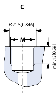
150-603.10-C
